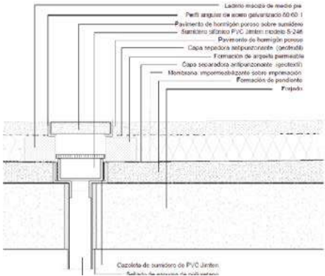
Detalle del registro sumidero en cubierta transitable
