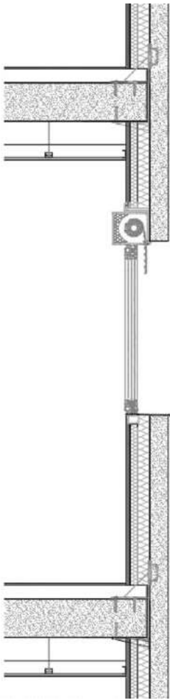
Sección
